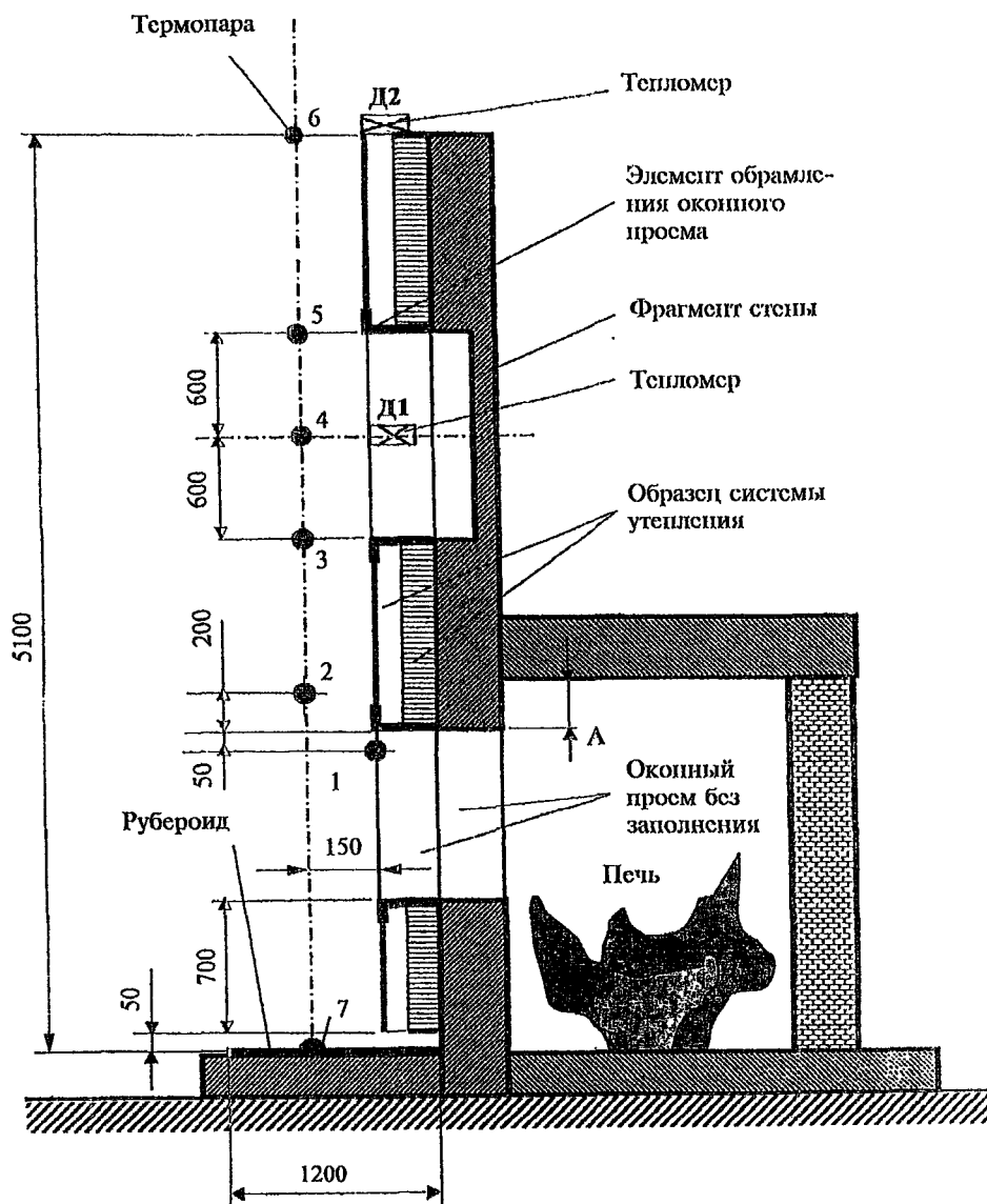
Рисунок 2б. Схема установки с образцом системы утепления Разрез I - I
