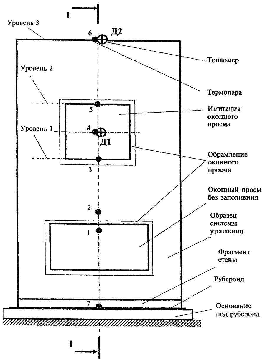
Рисунок 2а. Схема установки с образцом системы утепления Вид спереди
