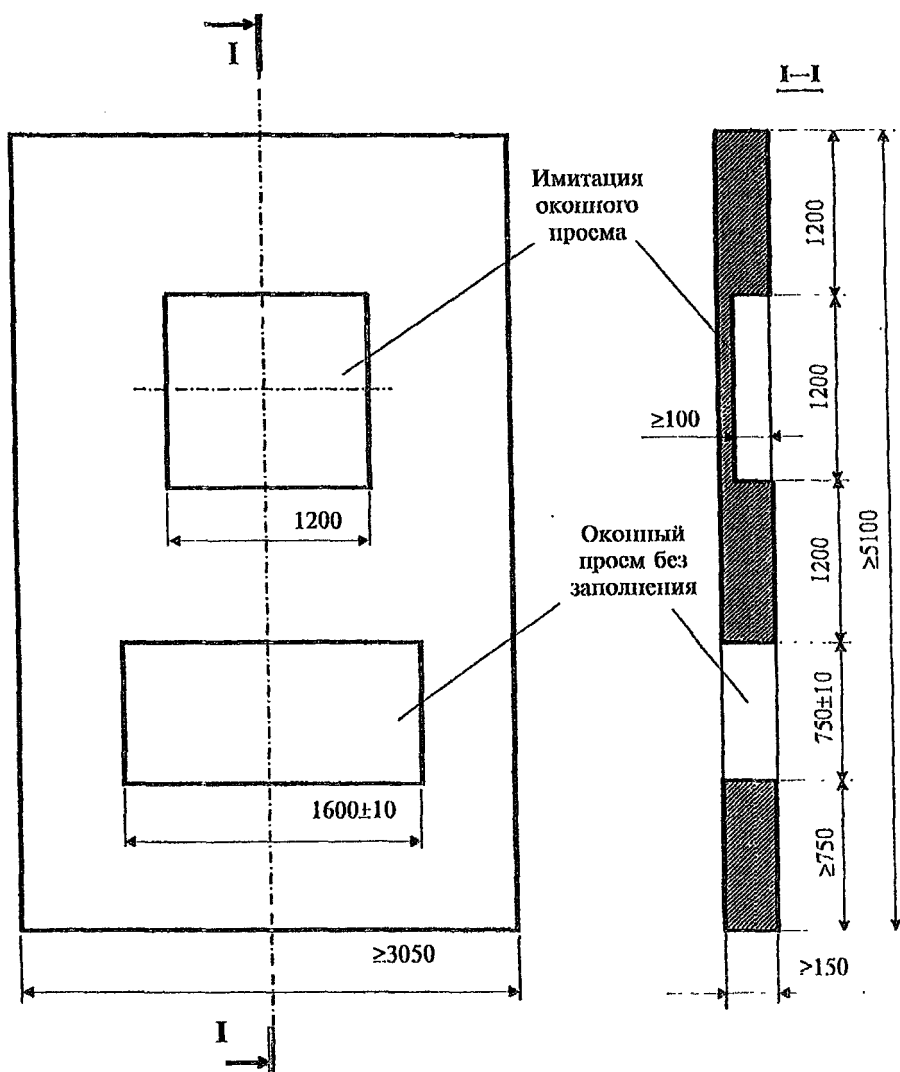
Рисунок 1. Фрагмент стены
